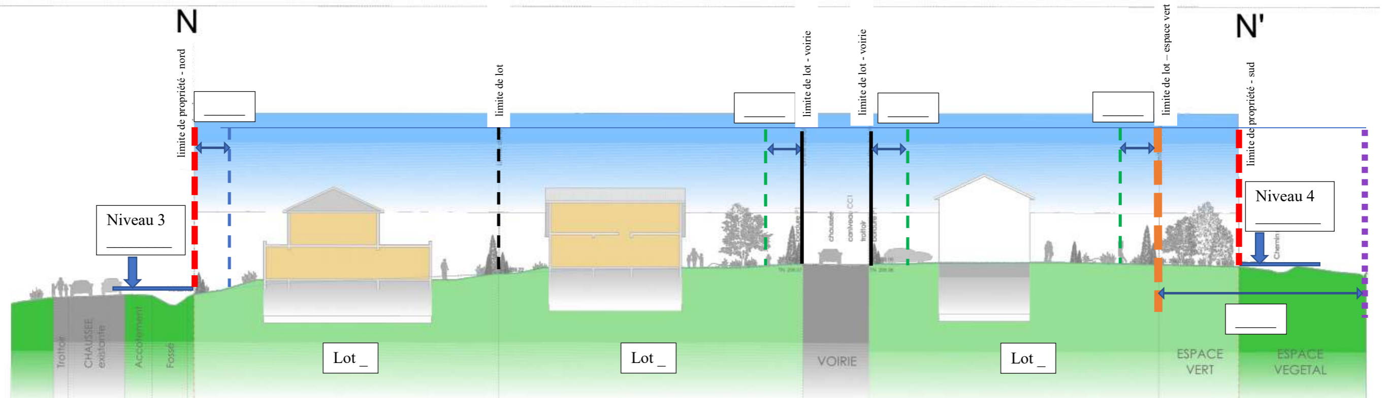
COUPES DE PRINCIPE MM' et NN'
